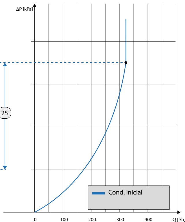
Curvas de funcionamento do circuito
