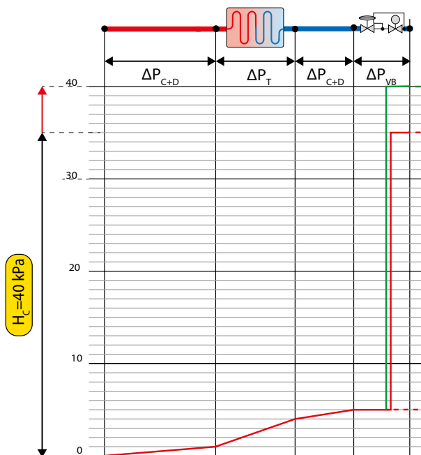
Gráfico de perdas de carga
