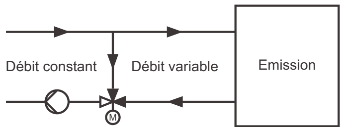
Vanne 3 voies montée en décharge inversée
