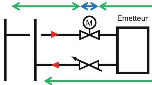
Détails du calcul de l'autorité pour une vanne deux voies
