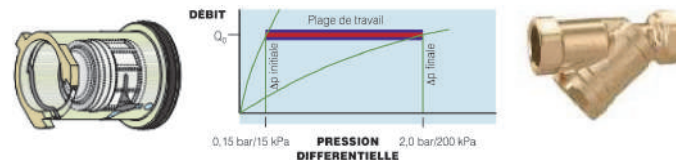
Vanne d'équilibrage dynamique (Caleffi)
