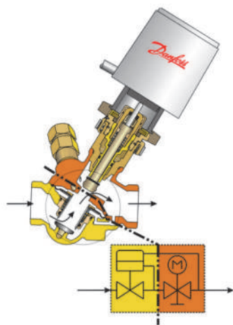
Représentation des deux principaux composants d'une vanne de régulation et d'équilibrage indépendante de la pression (Danfoss)
