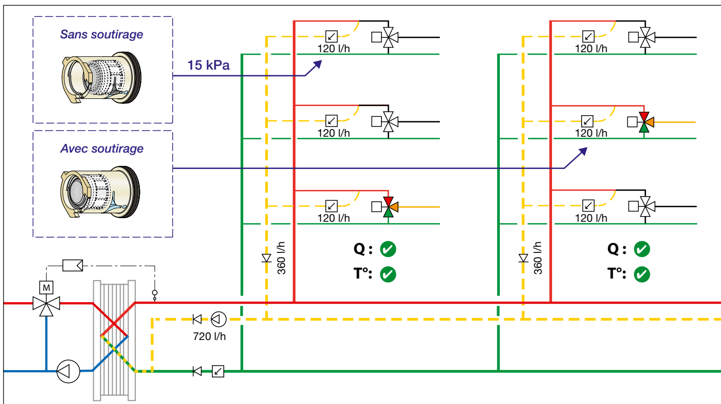
Le schéma ci-dessus présente une installation d'ECS avec bouclage équilibré à l'aide de vannes d'équilibrage automatique AUTOFLOW®
