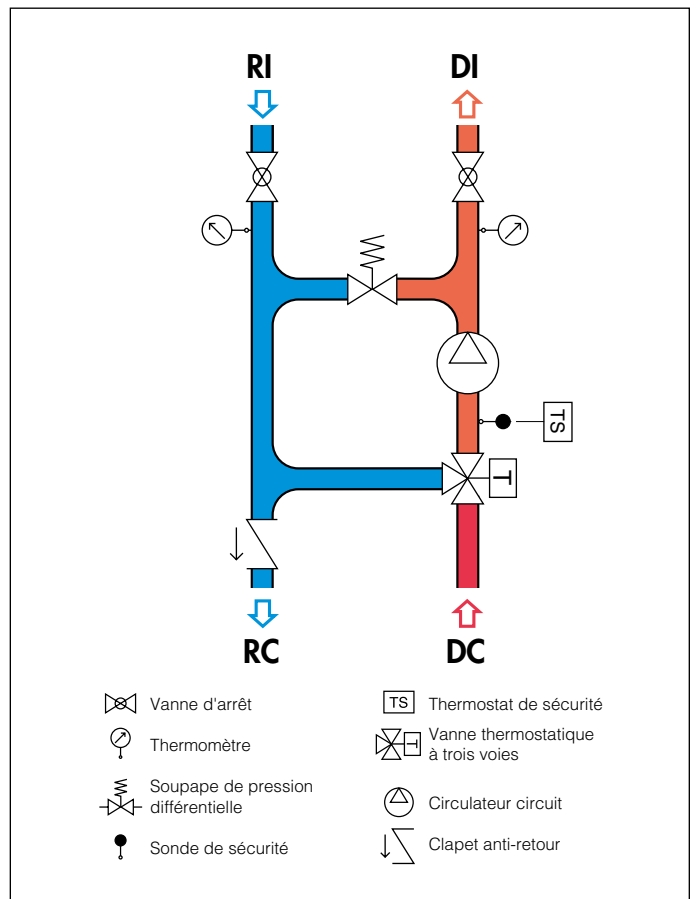
Schéma de fonctionnement hydraulique série 166
