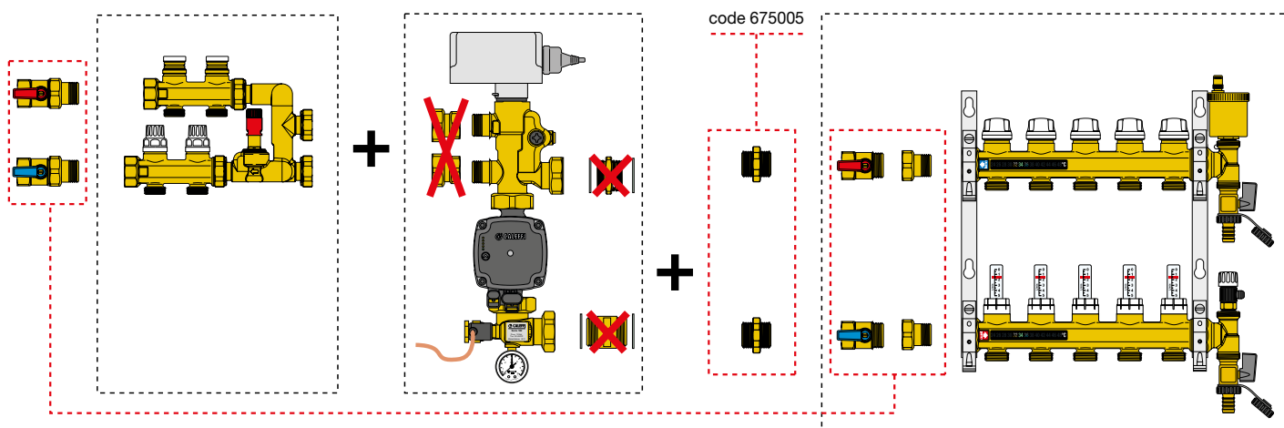
Composition du GRM série 181 avec collecteurs basse température série 664 et collecteurs haute température série 662
