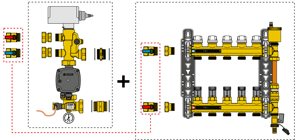
Composition du GRM série 181 avec collecteurs basse température série 662
