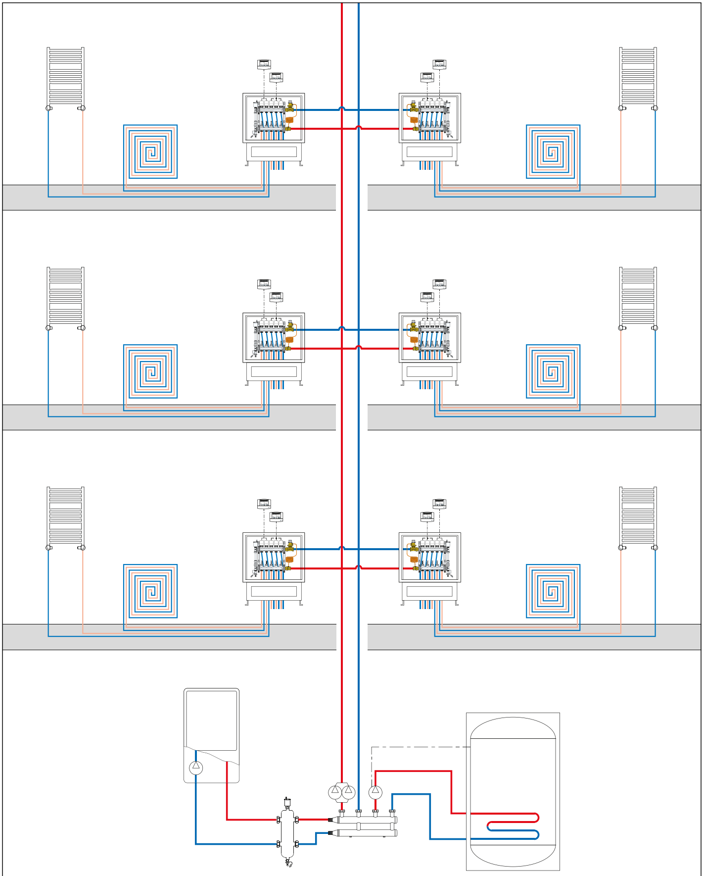
Schéma d'application du régulateur de pression différentielle série 140
