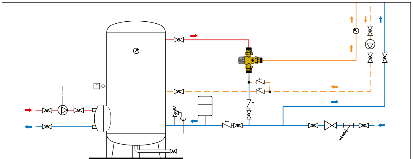
Schéma d'application du mitigeur série 5231
