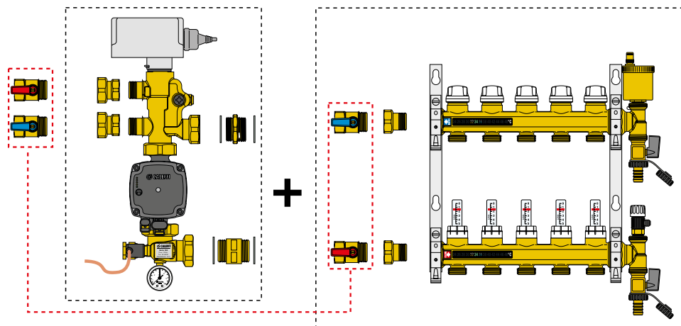
Composition du GRM série 181 avec collecteurs basse température série 664
