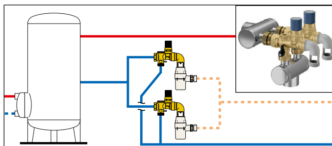
Schéma d'utilisation code 650972 avec groupe code 526163
