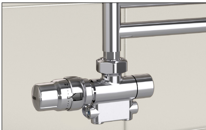
Exemple d'installation du robinet pour radiateur sèche serviette, plongeur vertical, modèle gauche, avec tête thermostatique.
