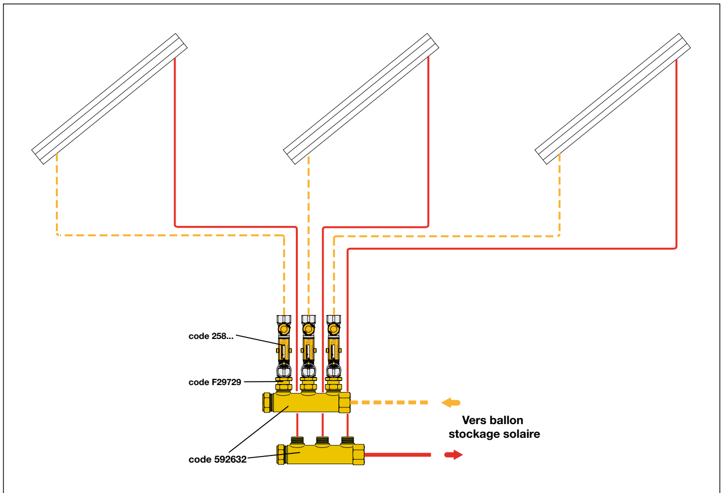
Schéma d'application pour l'équilibrage de 3 champs de capteurs solaires
