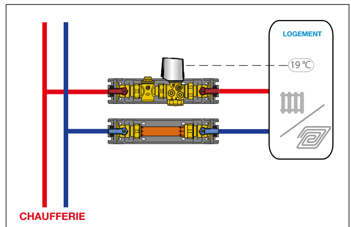
Schéma d'application
