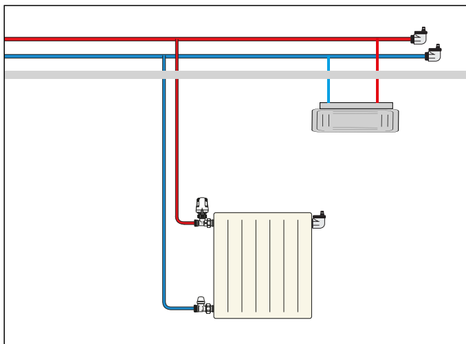
Schéma d'application AERCAL®
