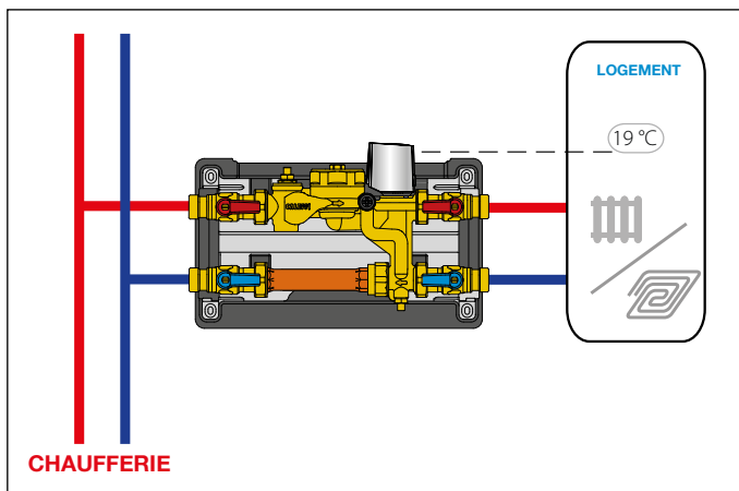
Schéma d'application
