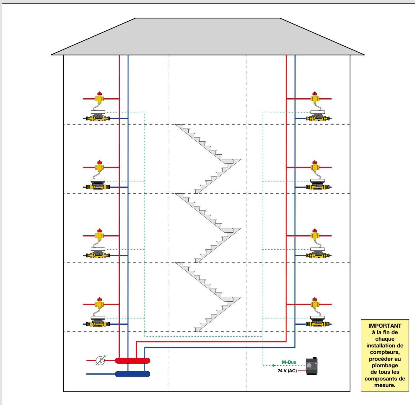
Schéma d'installation avec comptabilisation sur chaque dérivation
