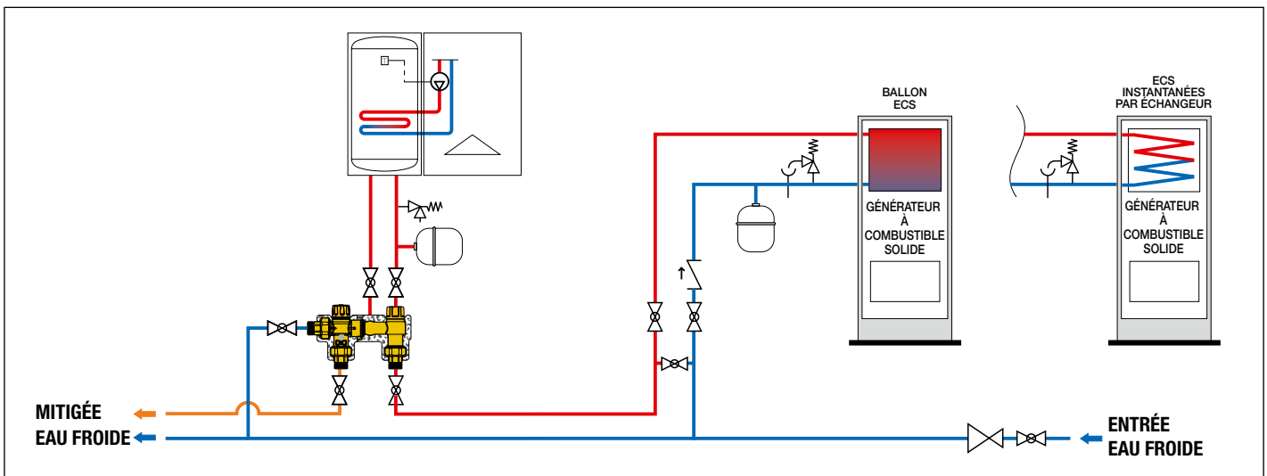
Schéma d'application kit SOLARINCAL-T série 262 avec générateur à combustible solide
