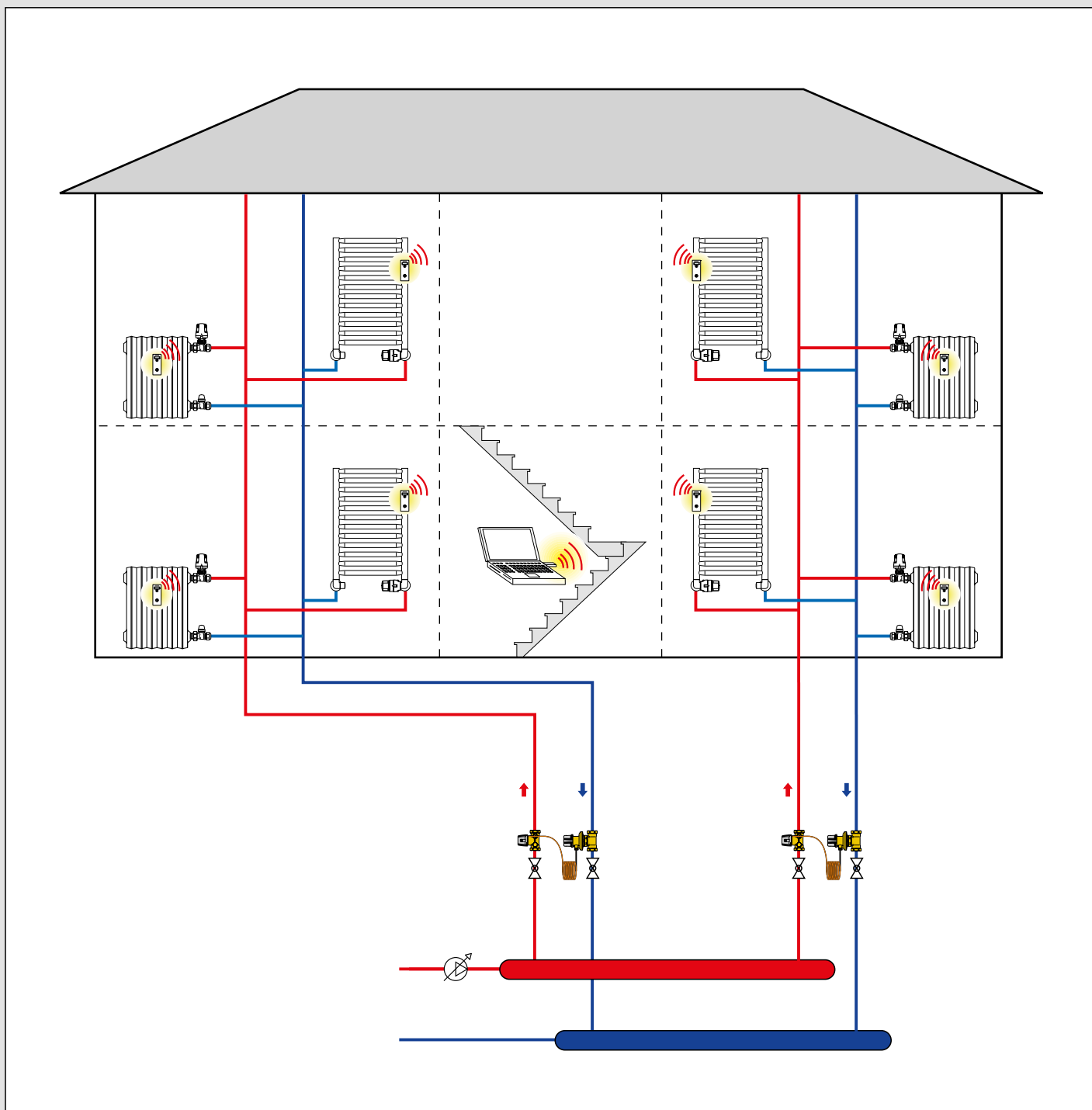
Schéma indicatif d'installation
