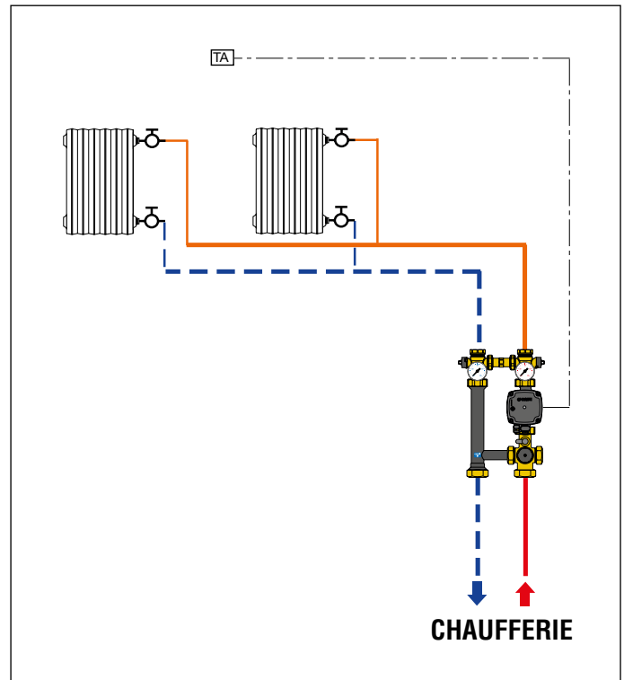
Schéma d'application groupe de régulation motorisé série 166
