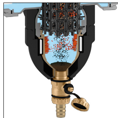
Filtration des particules ferreuses
