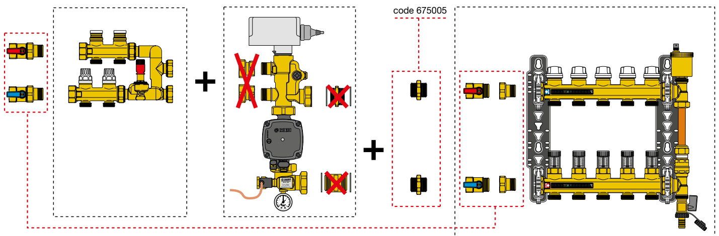
Composition du GRM série 181 avec collecteurs basse température série 662 et collecteurs haute température série 662
