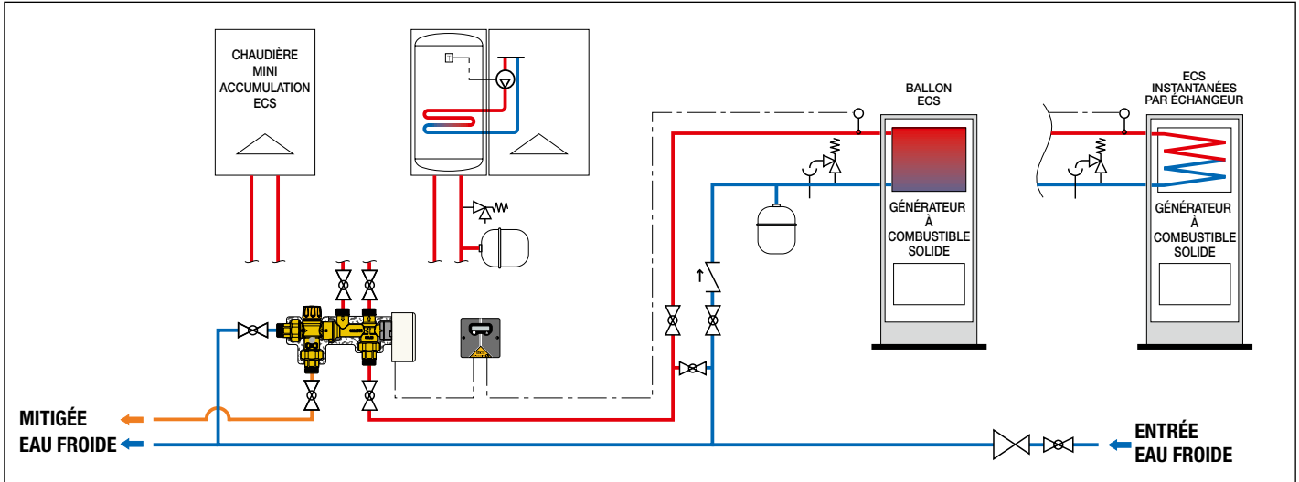
Schéma d'application kit SOLARINCAL série 265 avec générateur à combustible solide
