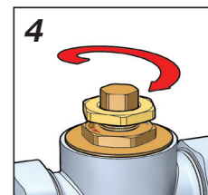
Bloccaggio regolazione con ghiera
