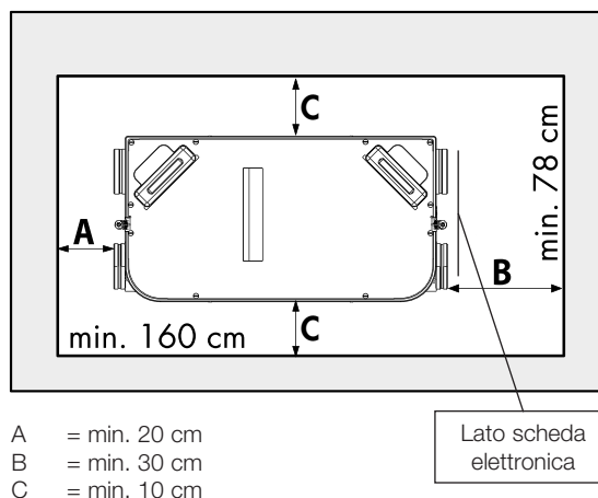
Dimensioni botola di ispezione
