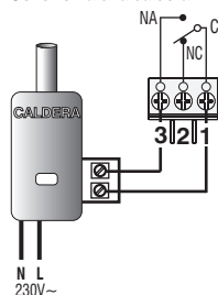
Conexión a una caldera
