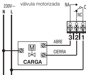
Conexión a una válvula motorizada
