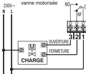
Raccordement à une vanne motorisée
