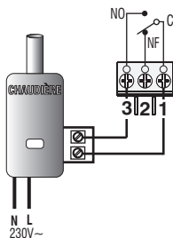
Raccordement à une chaudière
