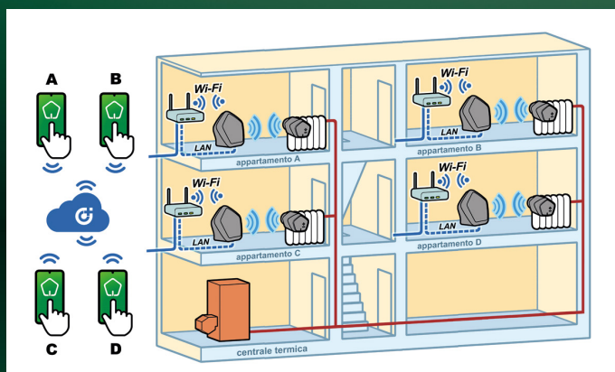
Toepassingsvoorbeeld: regeling in een centrale verwarmingsinstallatie met stijgleidingen.
