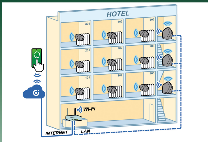
Toepassingsvoorbeeld: regeling in middelgrote tot grote installaties
