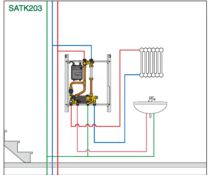
Radyatör Sistem
