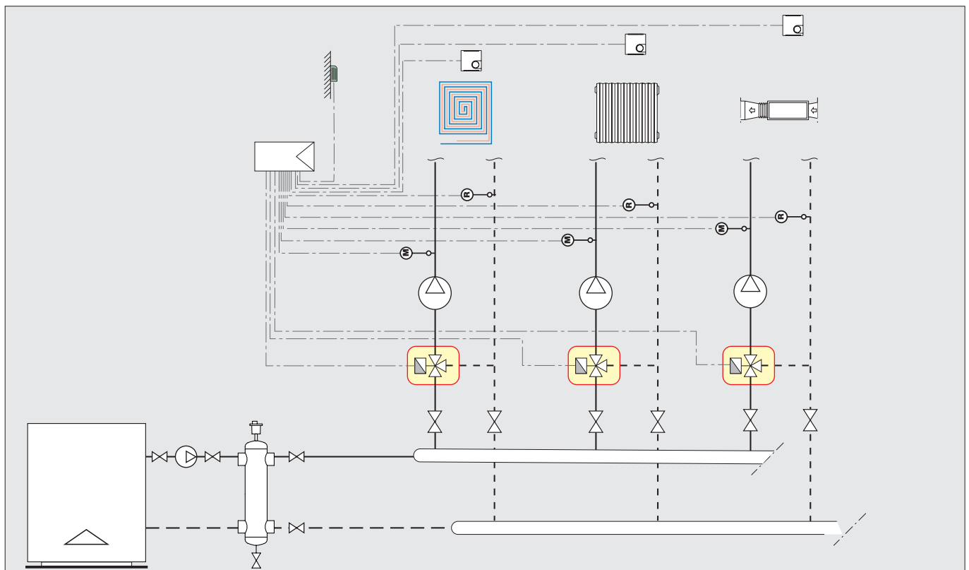
Valvola miscelatrice
