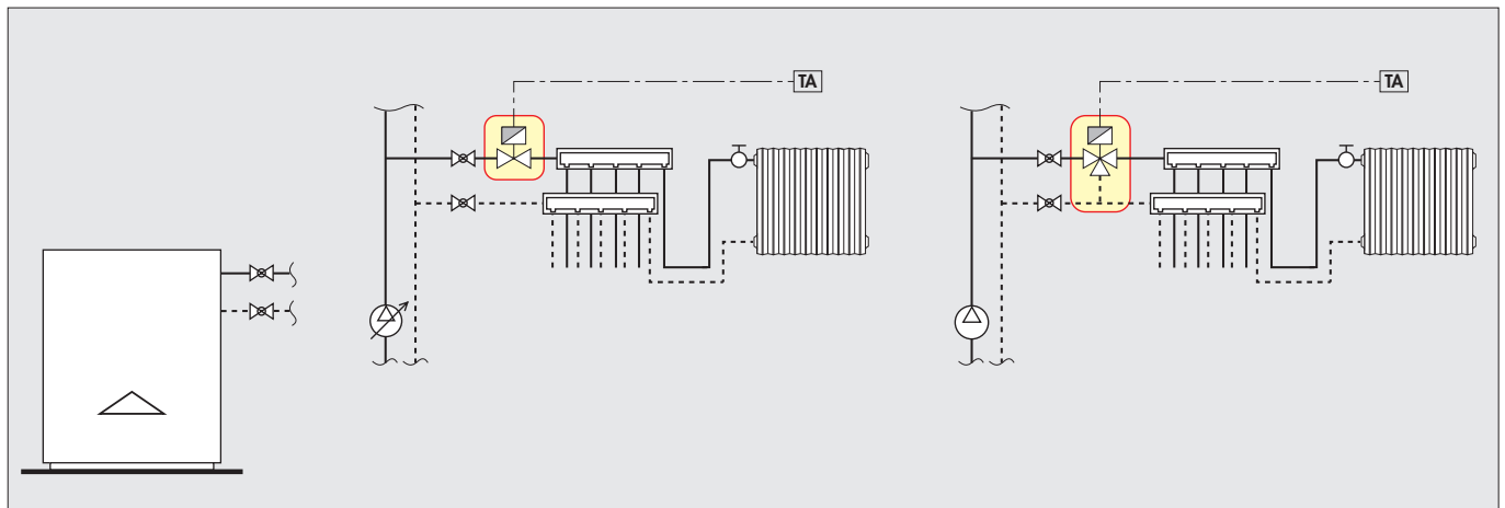
Valvola deviatrice
