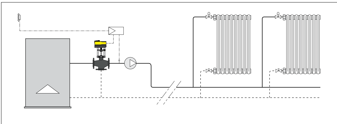
Regulacja pogodowa za pomocą zaworu trójdrożnego w instalacji centralnego ogrzewania z grzejnikami.
