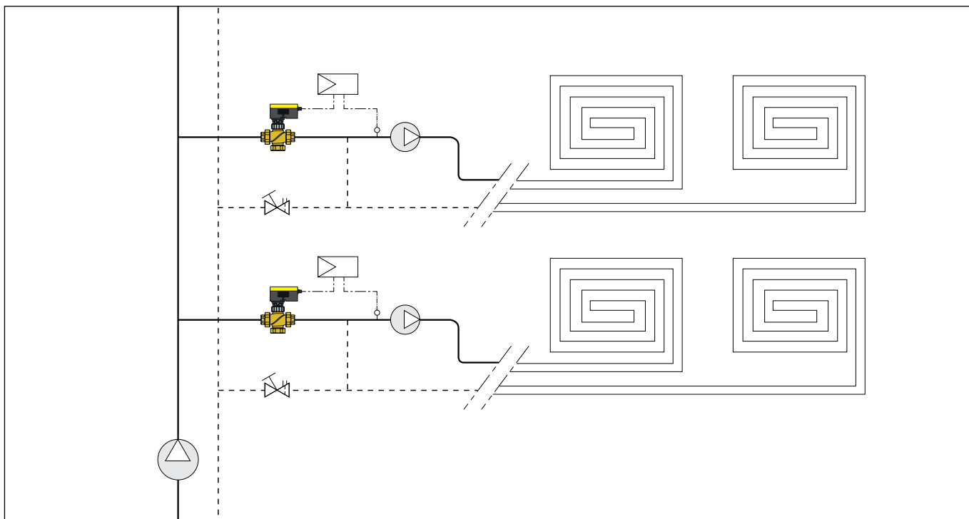
Regulacja temperatury za pomocą zaworów dwudrożnych w instalacjach z ogrzewaniem podłogowym.
