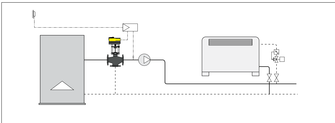
Regulacja pogodowa za pomocą zaworu trójdrożnego w instalacji centralnego ogrzewania.
