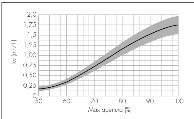
Kv vs. apertura max motore - primario riscaldamento
