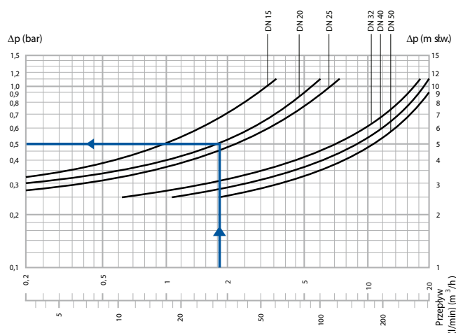
Wykres 2 (Spadek ciśnienia)
