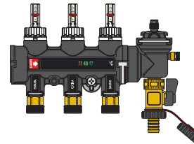
Kopfgruppen mit automatischem Schnellentlüfter und Füll-/Entleerungshahn
