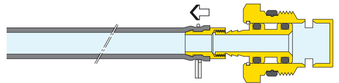
Zawór otwarty
