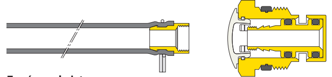
Zawór zamknięty
