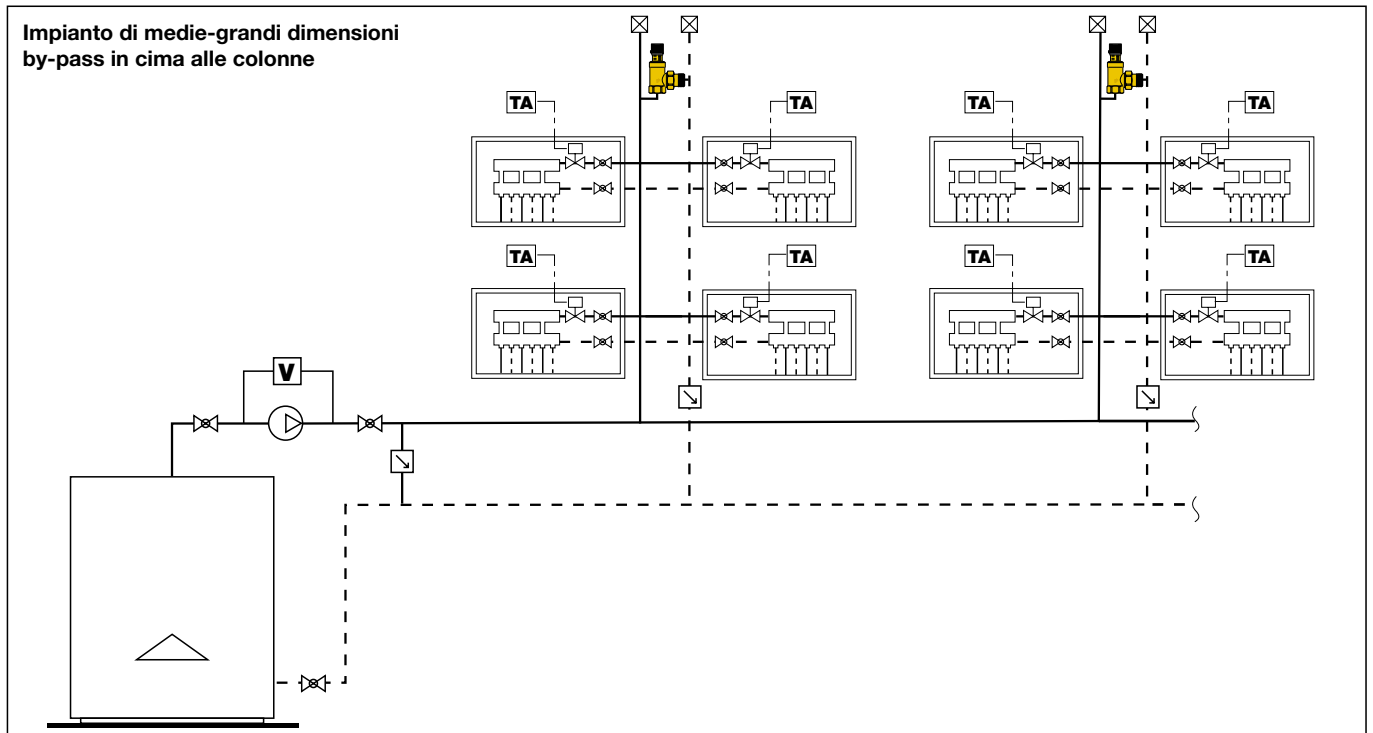
Impianto a pompa di calore by-pass in centrale
