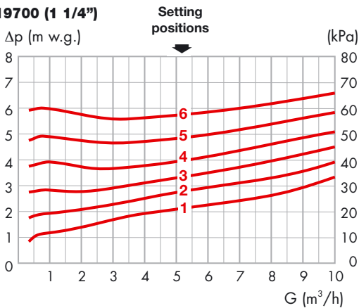
cod. 519700 (1 1/4")
